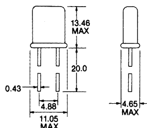
HC49U
