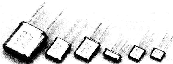
HC-33/U HC-18/U HC-49/U HC-49/S UM-1 UM-5
