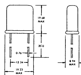
HC33U
